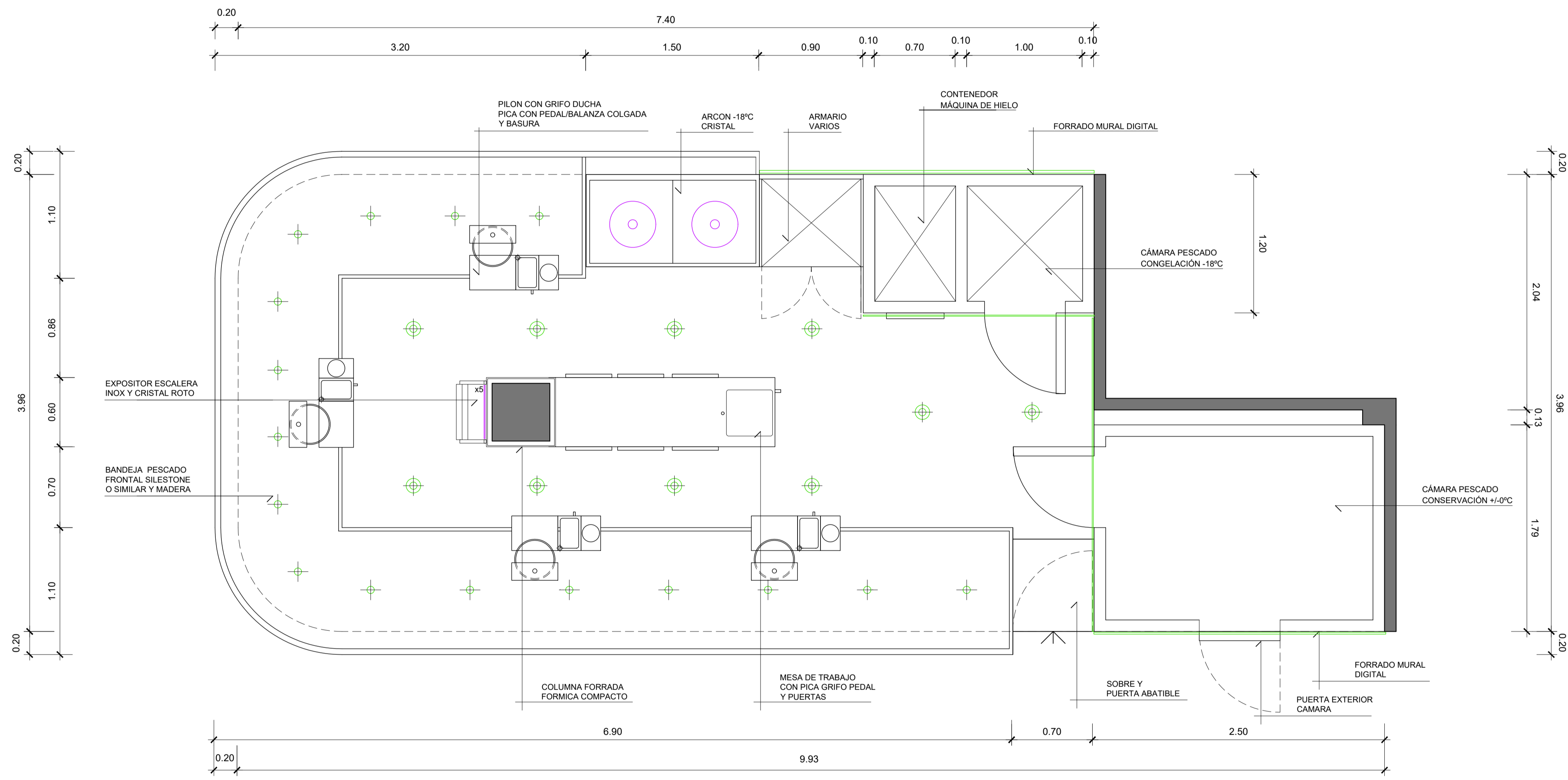
PLANTA DISTRIBUCIÓN E ILUMINACIÓN
