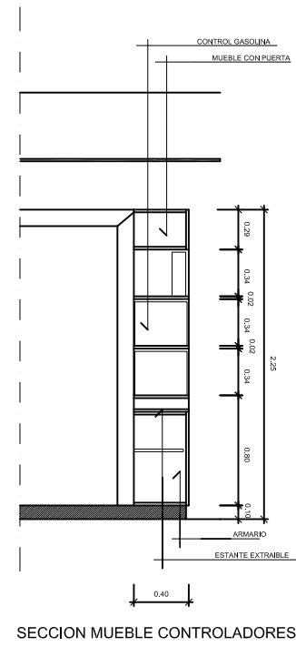
SECCION MUEBLE CONTROLADORES
