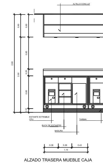
ALZADO TRASERA MUEBLE CAJA
