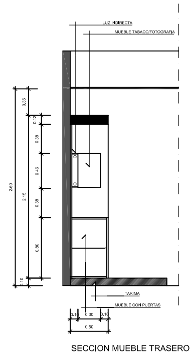
SECCION MUEBLE TRASERO
