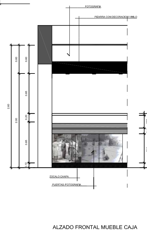
ALZADO FRONTAL MUEBLE CAJA
