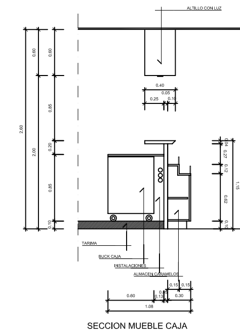
SECCION MUEBLE CAJA
