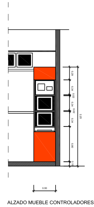
ALZADO MUEBLE CONTROLADORES
