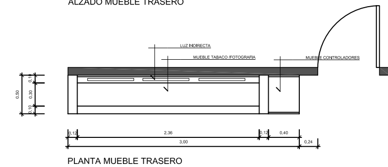
PLANTA MUEBLE TRASERO
