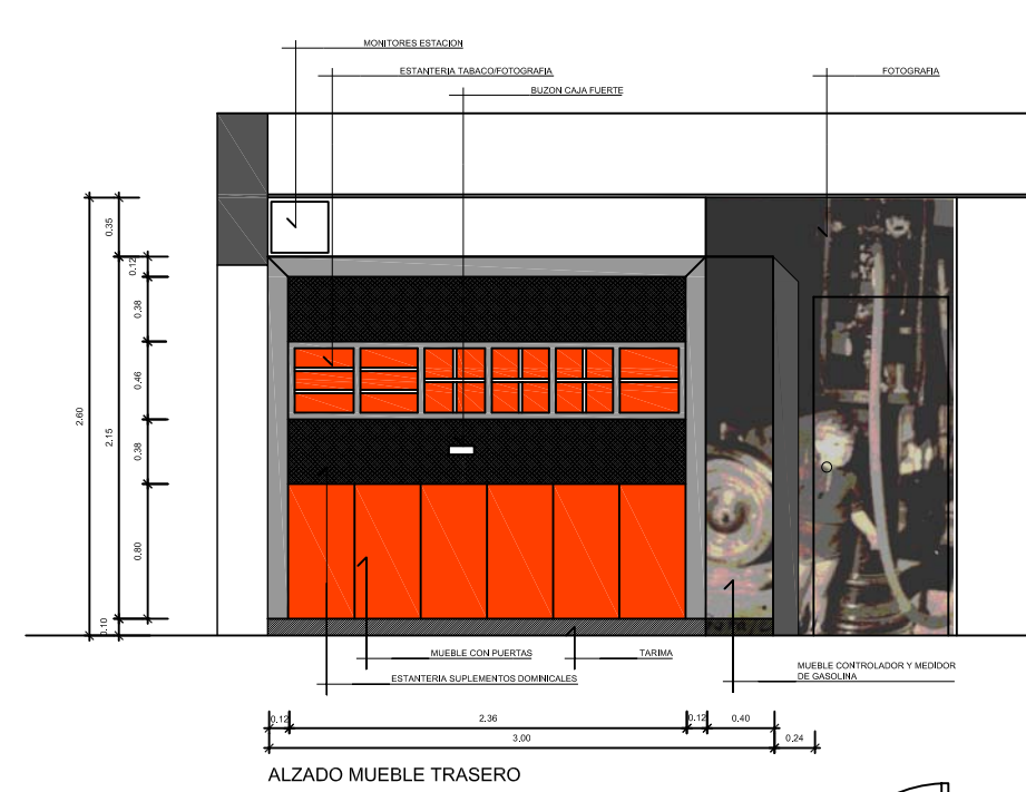
ALZADO MUEBLE TRASERO
